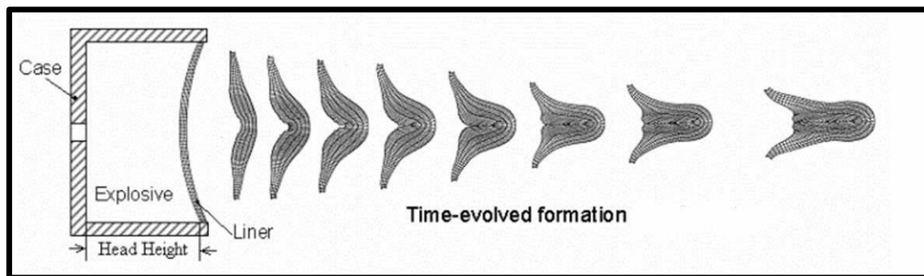
Figura 51 (U) Diseño genérico de una ojiva penetrante formada por explosión
